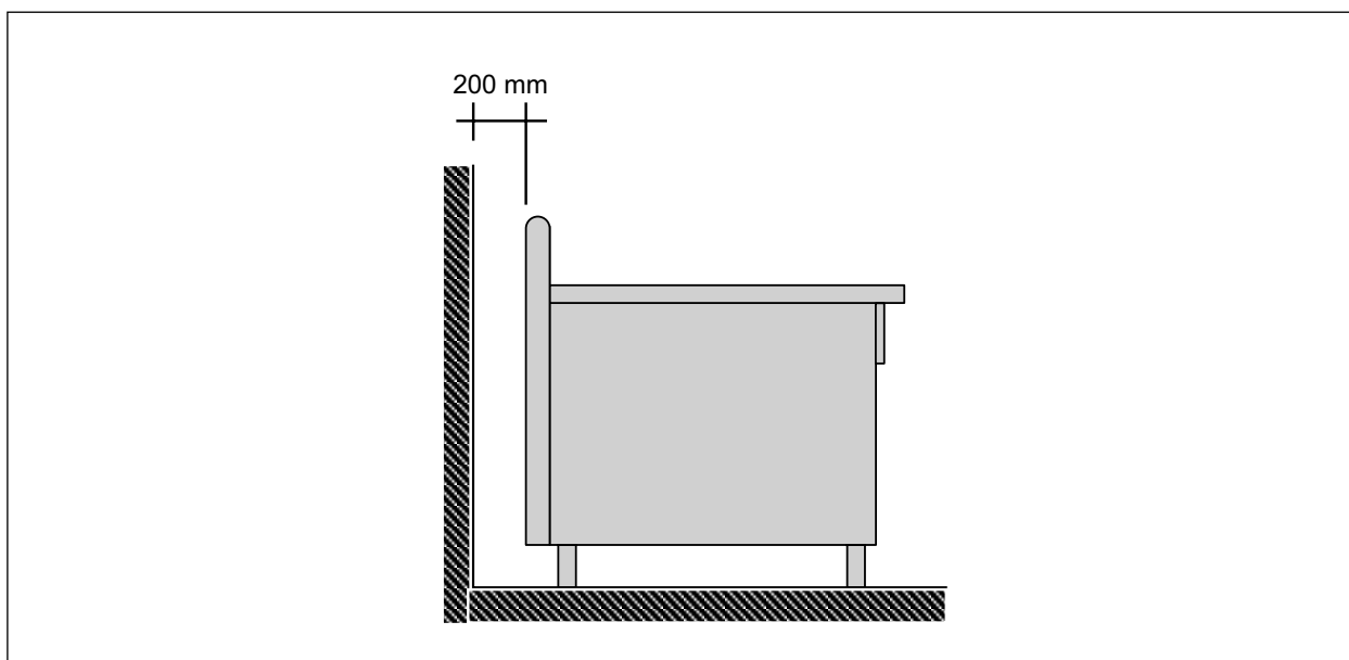
Fig. 21 Distanza minima da pareti infiammabili
