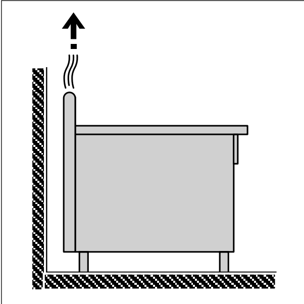
Fig. 23 Scarico calore
