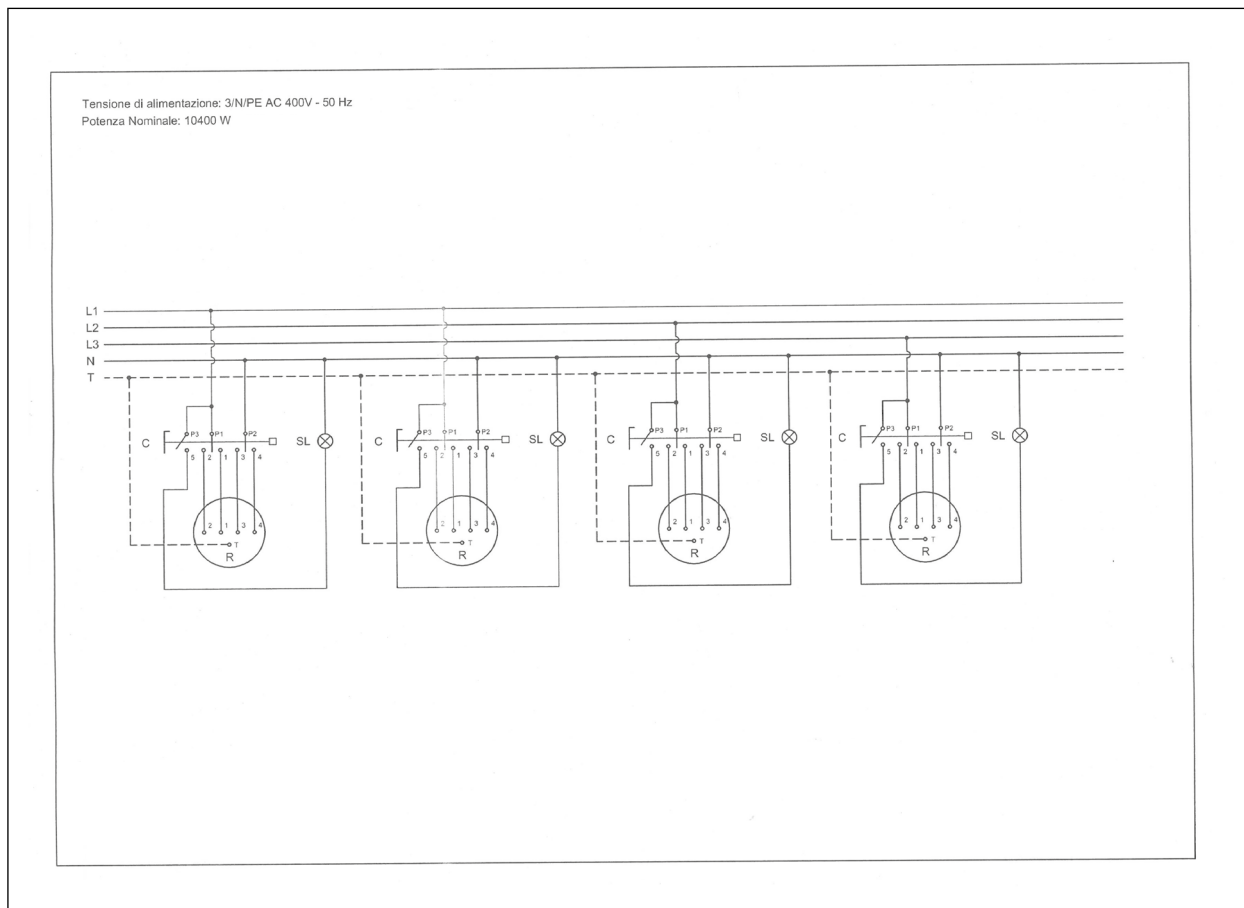
Fig. 25 Schema elettrico 1
