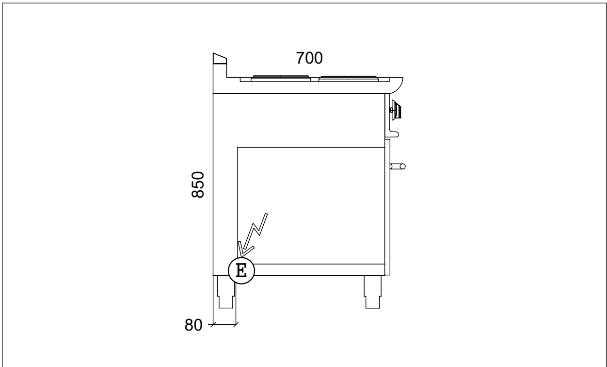
Fig. 17 Dimensioni cucina con vano chiuso o forno
