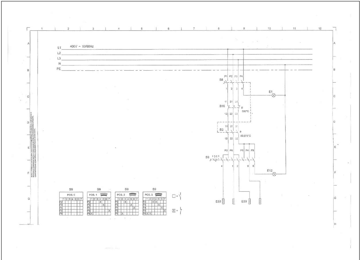
Fig. 26 Schema elettrico 2 - Forno elettrico
