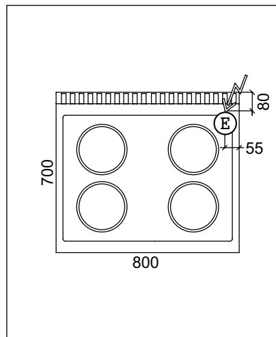
Fig. 15 Cucina 4 piastre
