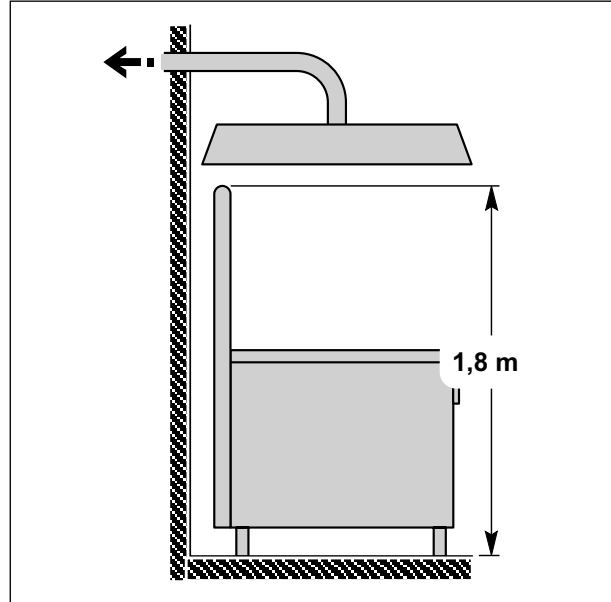
Fig. 24 Scarico attraverso cappa
