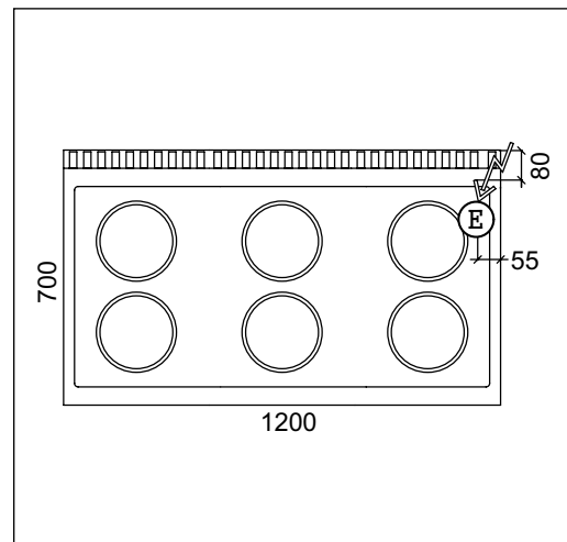
Fig. 16 Cucina 6 piastre
